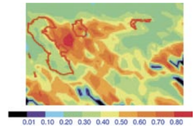
Рис. 13. Средняя оптическая толщина атмосферных аэрозолей на длине волны 550 \text{ нм} за апрель – май 2001 г. и 2002 г. (спутник NASA [ 2 ])
