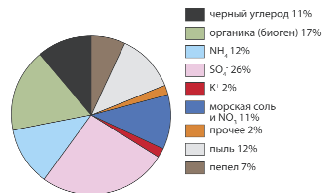
Рис. 2. Относительный вклад различных химических составляющих в аэрозольную оптическую толщину [3]
