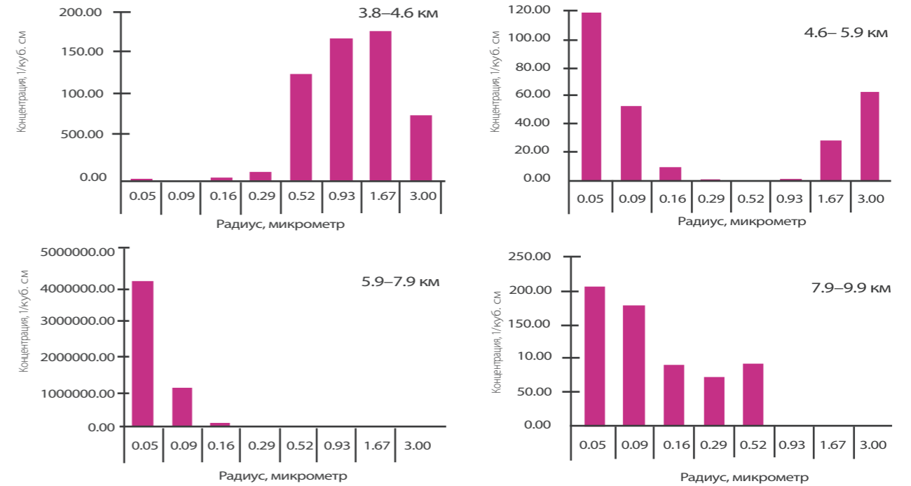
Рис. 10. Распределения концентраций частиц по размерам в различных слоях пыли и облака [5]
