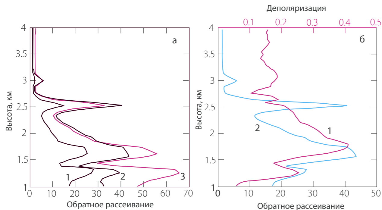
Рис. 12. Вертикальные профили отношения рассеяния R(h) (а) на трех длинах волн: 1 - \lambda=355 \text{ нм} , 2 - \lambda=532 \text{ нм} , 3 - \lambda=1064 \text{ нм} ; совмещенные кривые деполаризации D (1) и отношения рассеяния (2) на длине волны 532 \text{ нм} . Пыль. 03:56 ч 8.08.2003 г.[8]
